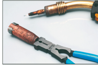
Nozülün ucundan lekelerin çıkarılması
