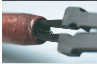
Nozülün içinden ve dışından lekelerin çıkarılması
