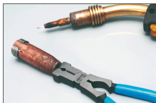
Čistenie koncovky tryskovej trubice
