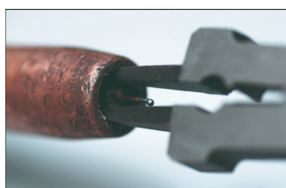
Удаление сварочных брызг изнутри и снаружи сопла
