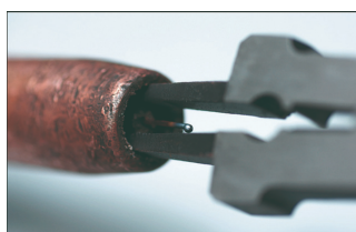
Удаление сварочных брызг изнутри и снаружи сопла
