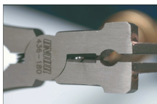
Вытягивание проволоки из сопла
