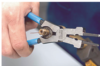
Снятие и установка втулки
