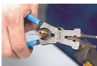
Demontare si montare a difuzorului izolant
