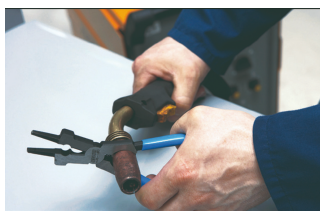
Demontare si remontare a duzei
