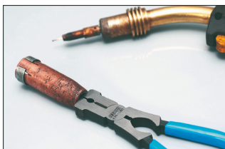
Usuwanie nagaru i odprysków z końcówki dyszy
