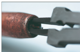
Usuwanie nagaru i odprysków z wnętrza i zewnętrznej części uchwytu
