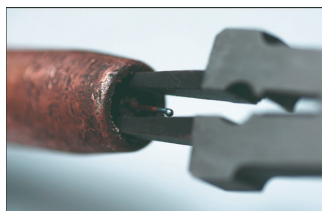
Rimozione delle scorie dall'estremità del bocchello
