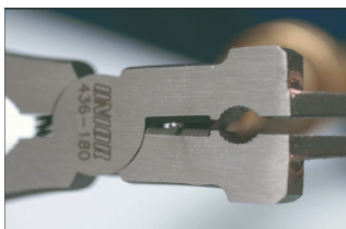
Corte de alambre
