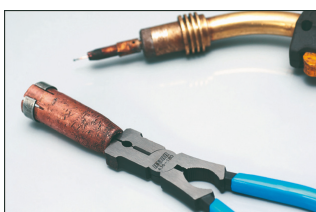
Remoción de salpicaduras de la parte final de la boquilla
