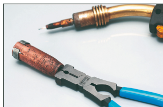
Čištění konce tryskové trubice
