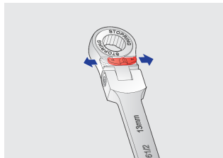
Carraca: funciona en ambos sentidos, el sentido de giro se puede cambiar con un botón.
