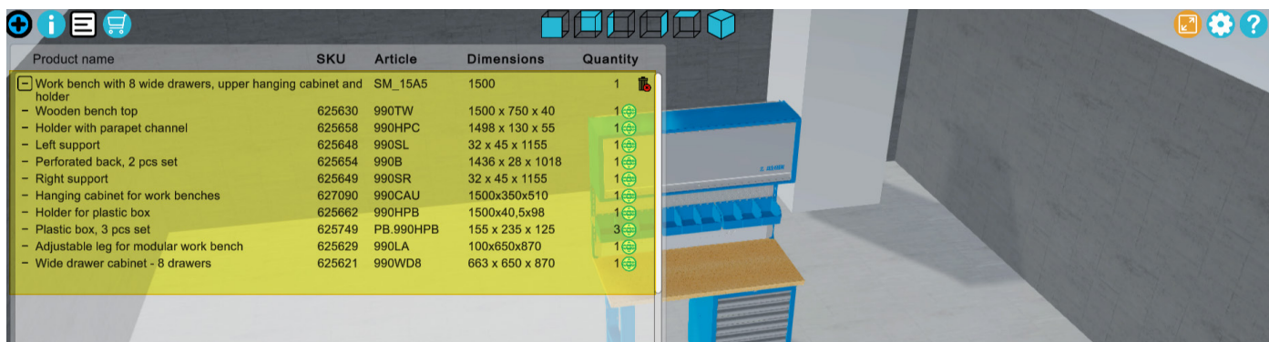
Montageliste aller hinzugefügten Elemente.
